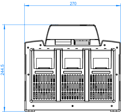
底视
