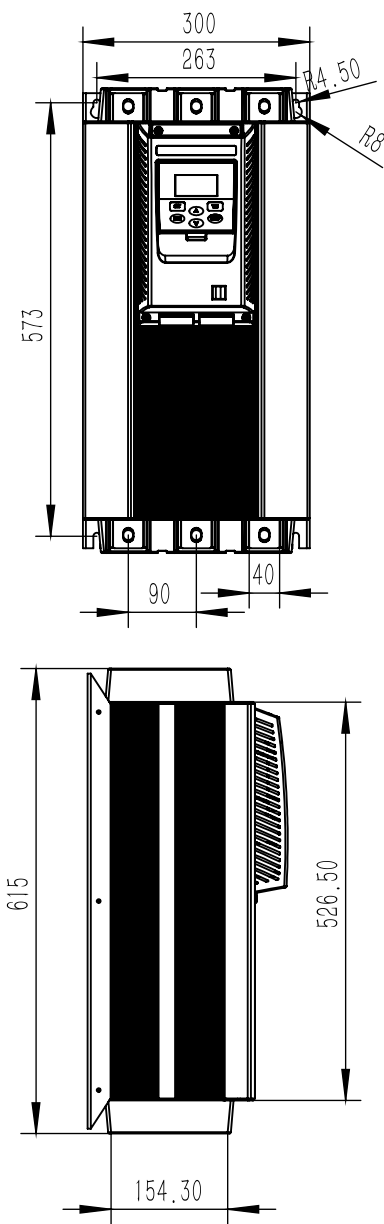
R5 尺寸详情
