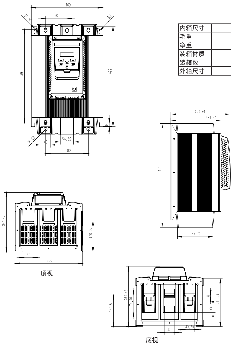
R4 尺寸详情
