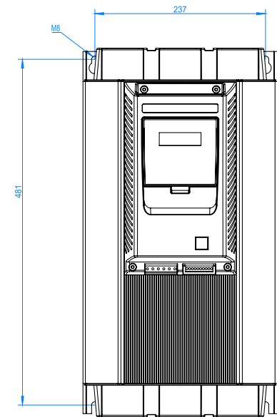
R3 尺寸详情
