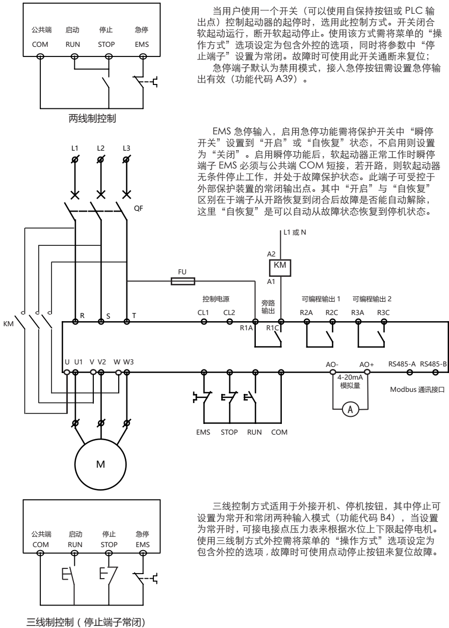
图 3-6 标准接线图
