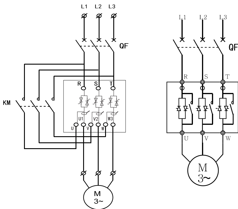
图 3-5 SJR3-2000P 基本线路连接
