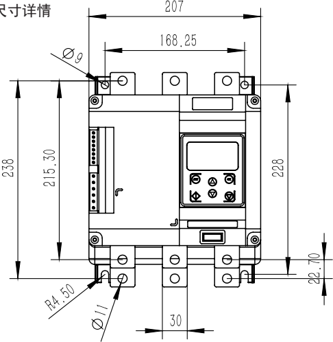
S1 尺寸详情
