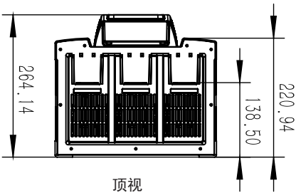
顶视
