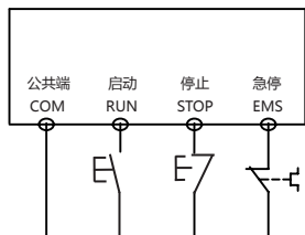
三线制控制（停止端子常闭）
