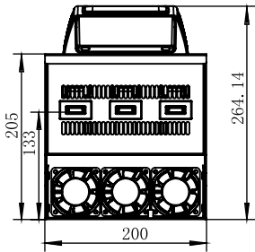
顶视
